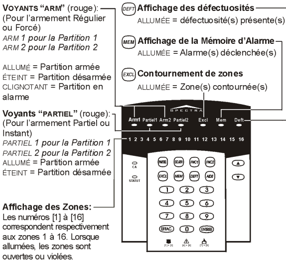
Figure 2.2: Vue d'ensemble du clavier à DEL 1689
